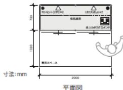
平面図
