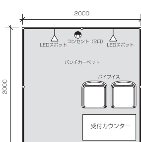
【平面図】
